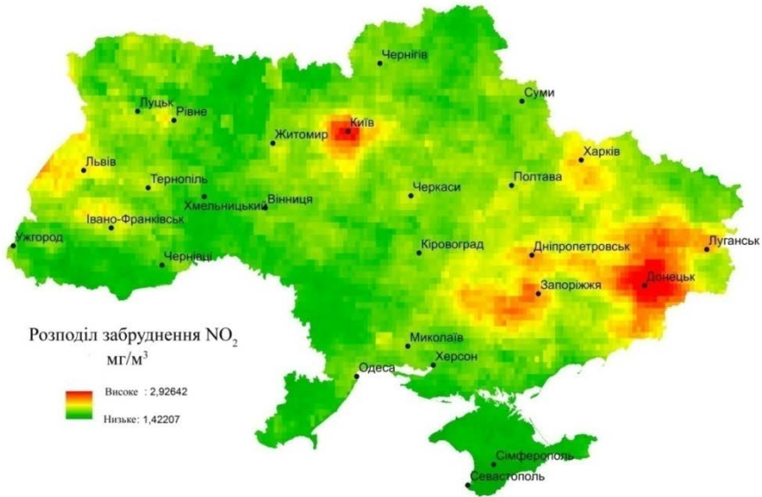
Рисунок 4 – Кореговані за інструментальними дослідження виміри забруднення NO 2
