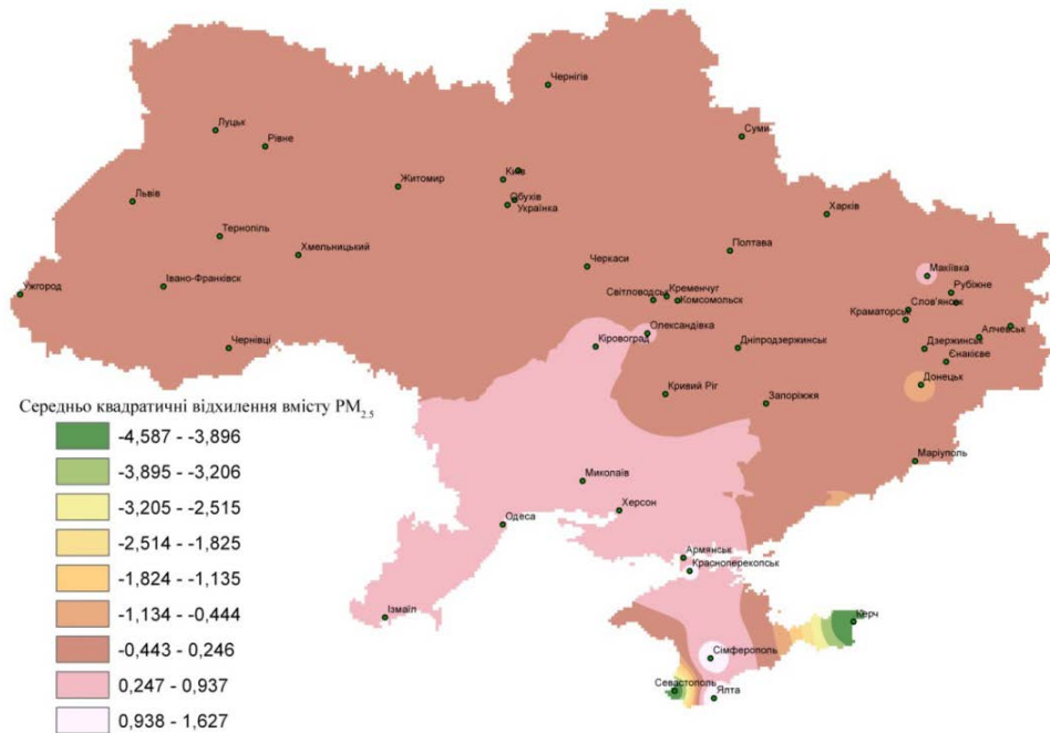
Рисунок 6 – Розподіл середньоквадратичних відхилень для географічно зваженої регресії PM_{2.5}
