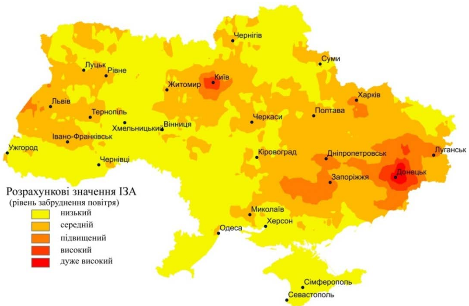
Рисуюнок 6 – Виміри ІЗА на основі супутникових даних
