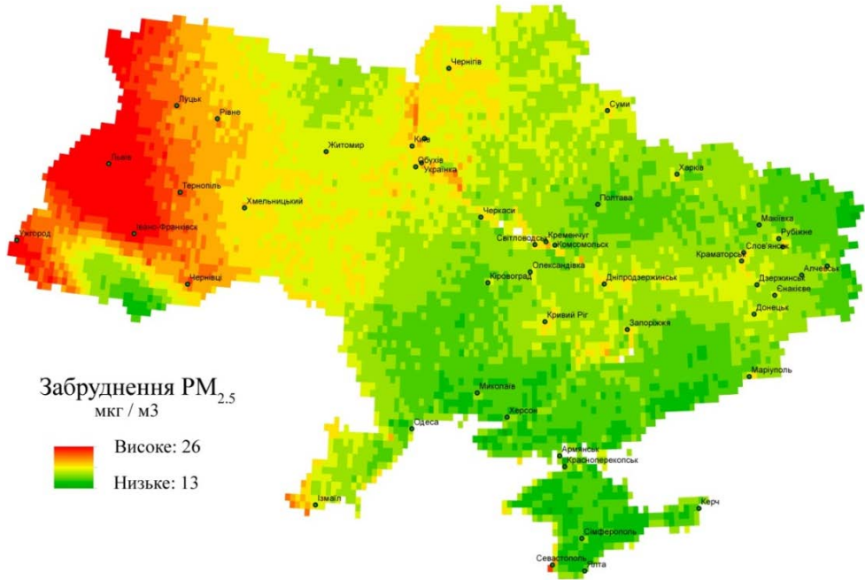
Рисунок 5 – Розподіл середньорічних значень PM_{2.5} на території України у 2012 р.
