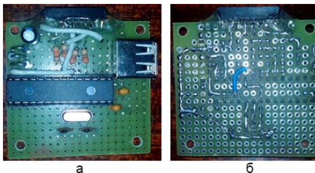
Рис. 3.17. Готовий пристрій
