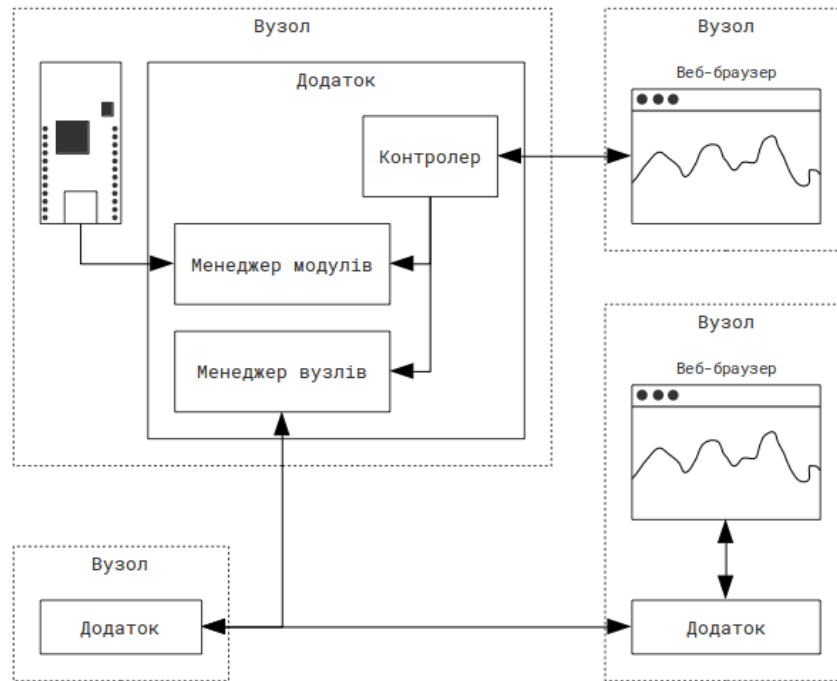
Рис. 3.25. Схема роботи третьої версії
