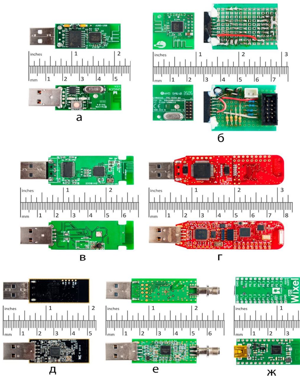
Рис. 1.8. Загальний вигляд плат аналізаторів спектра: а – Metageek Wi-Spy 2.4i; б – CYWUSB6935 (LPT); в – Wi-detector; г – TI eZ430-RF2500; д – Ubiquiti AirView2; е – Metageek Wi-Spy 2.4x і ж – Pololu Wixel
