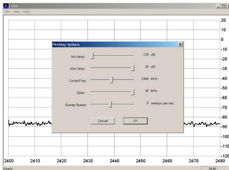
Рис. 3.19. Головні функції ПЗ LCSA
