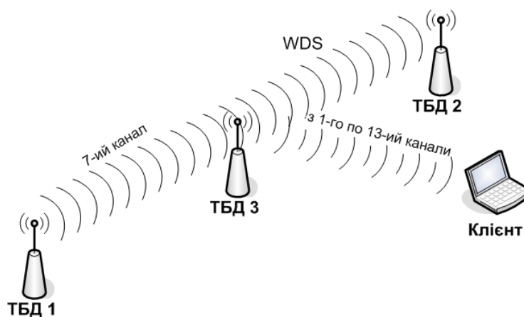
Рис. 3.1. Схема експерименту
