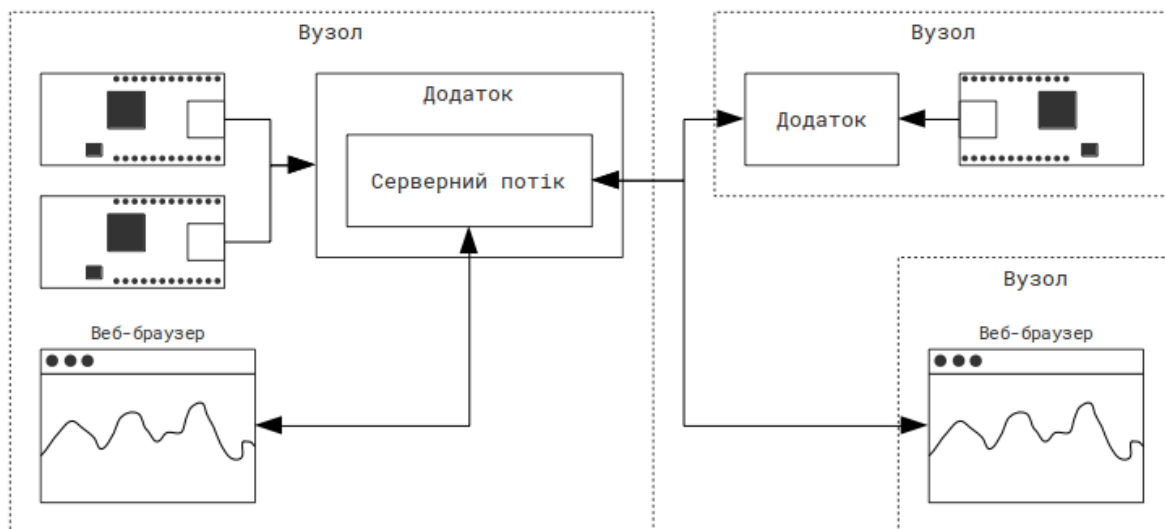
Рис. 3.24. Веб-інтерфейс першої версії системи моніторингу
