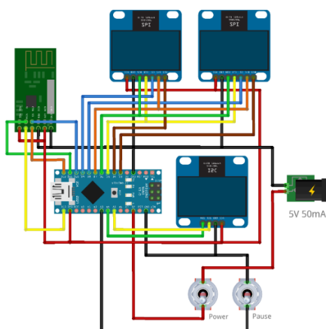
Рис. 2.5. Принципова схема розділеного приймача і блоку управління
