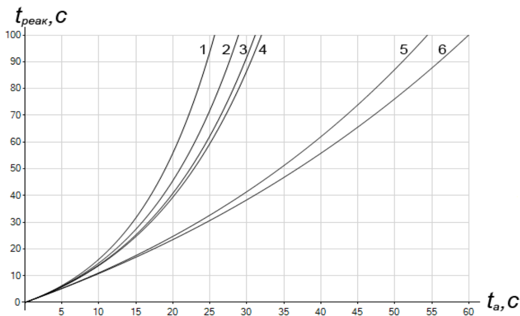
Рис. 1.4. Залежність ймовірності реалізації атаки від часу:
