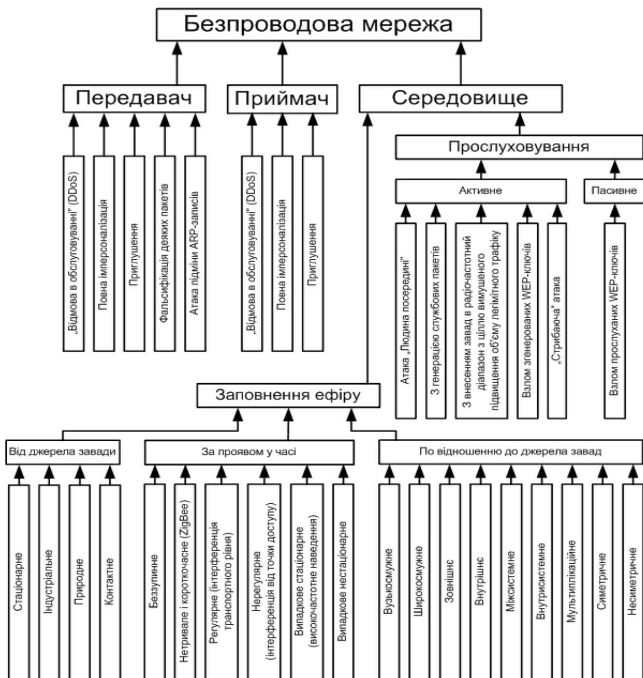
Рис. 1.2. Дерево атак на безпроводову мережу
