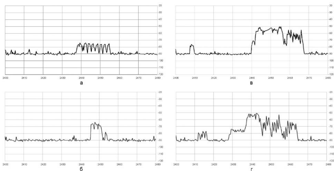
Рис. 3.10. Аналіз спектру, отриманого від Chirson CC2500: а – без використання антени і екрану; б – з використанням екрану, але без антени; в – з використанням антени, але без екрану; г – з використанням антени і екрану
