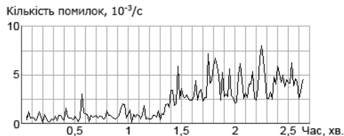
Рис. 3.5. Оцінка електромагнітної сумісності мереж на однакових частотах для 802.11g і 802.15.1
