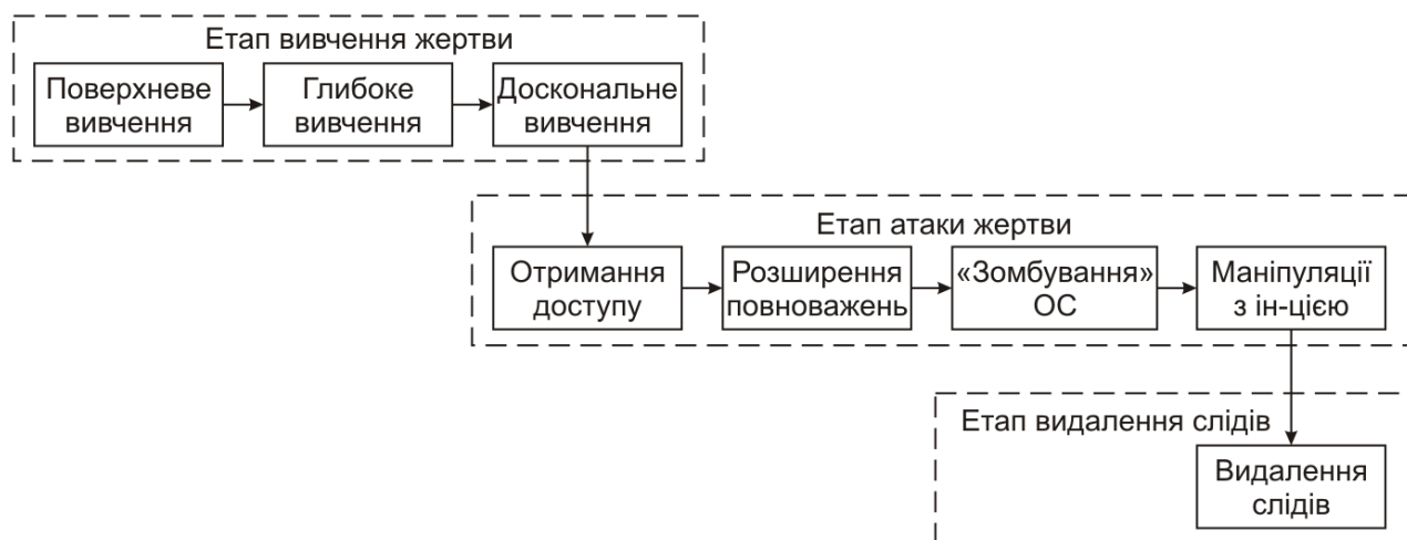
Рис. 1.6. Етапи моделі «зомбування»
