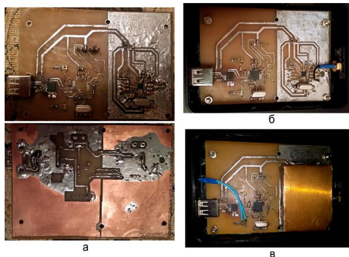
Рис. 3.9. Прототип аналізатора спектру на Chirson CC2500: а – із змонтованими елементами; б – встановлена в корпус; в – з припаяним екраном
