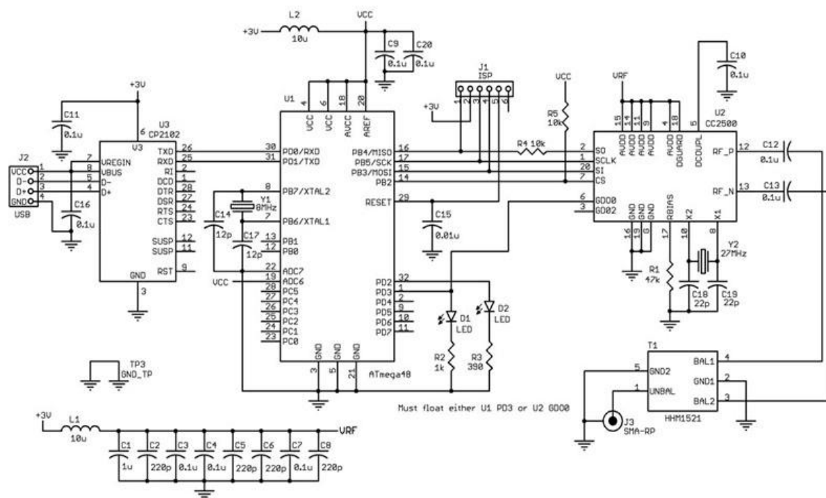
Рис. 3.6. Електрична принципова схема аналізатора спектру на Chirson CC2500
