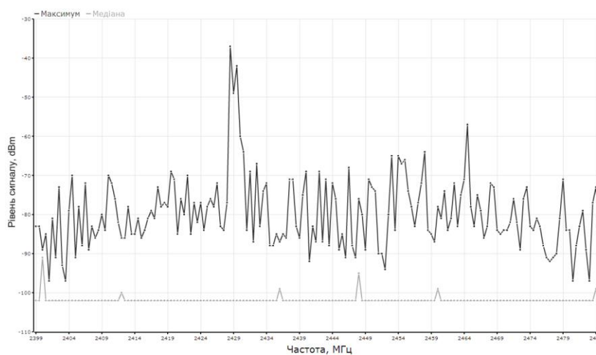
Рис. 1.19. Розподілення частот для двох каналів зі слабкими сигналами
