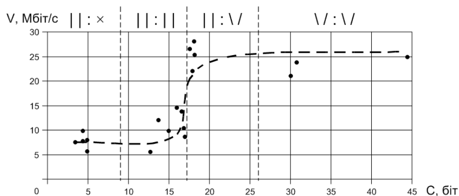
Рис. 3.41. Відношення інформаційної швидкості до пропускної здатності
