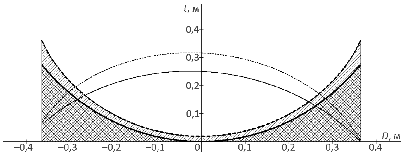
Рис. 2.14. Профілі ПЛ: класичної (суцільна лінія) і з усередненням (пунктирна), а також ФР в розкритті
