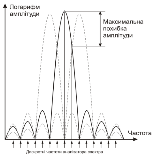
Рис. 1.9. Виникнення максимальної похибки при вимірюванні
