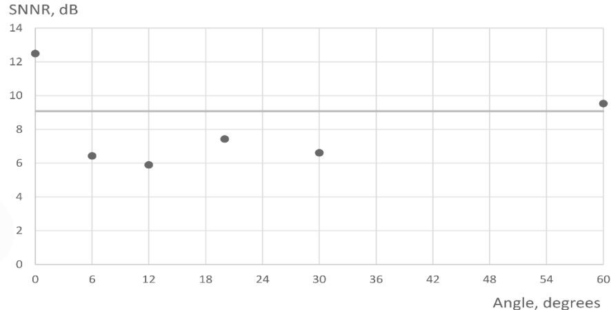
Рис. 3.36. Розподіл SNNR за кутовими напрямками
