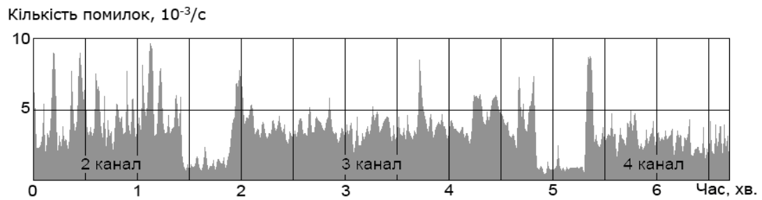
Рис. 3.3. Оцінка електромагнітної сумісності мереж на близьких частотах
