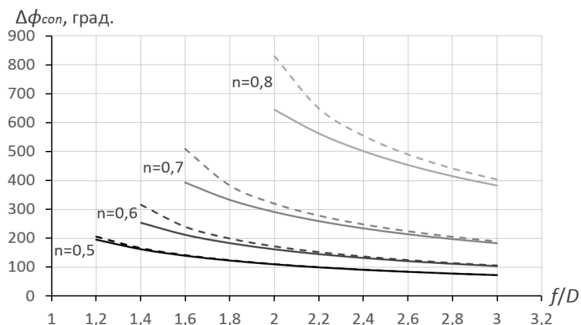
Рис. 3.40. Максимум увігнутості ФР
