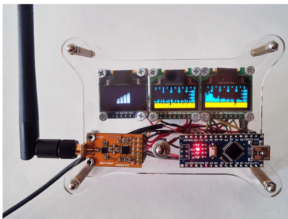
Рис. 2.6. Відокремлений приймач із зовнішньою антеною і блоком управління
