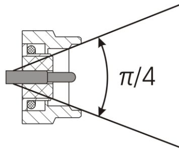
Рис. 2.18. Кут випромінювання SMA-роз'єму
