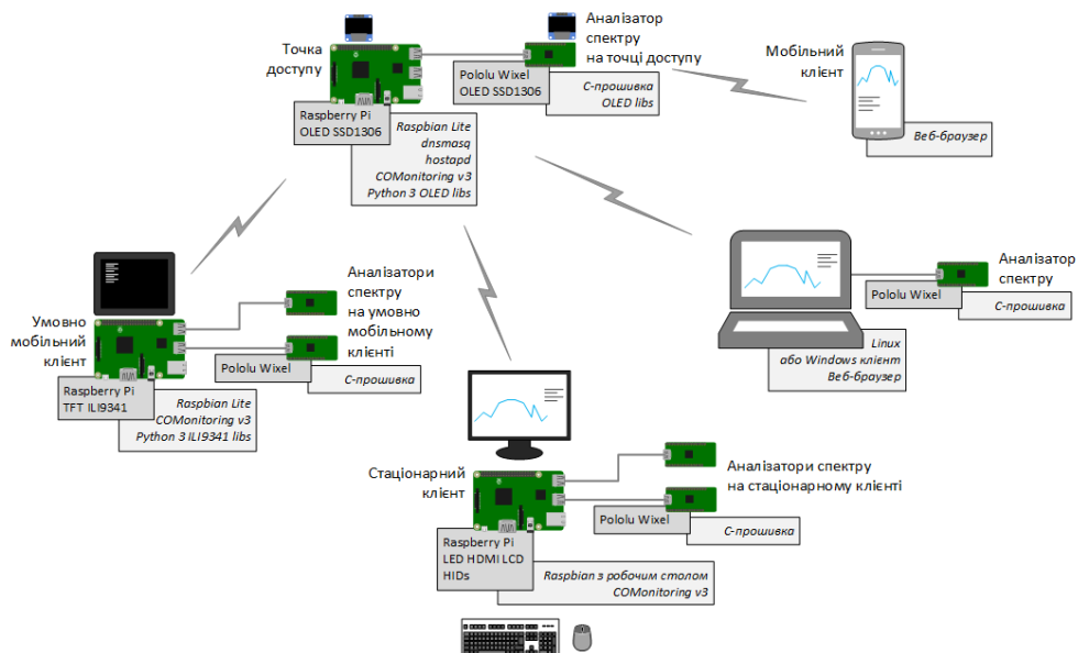
Рис. 2.11. Інфраструктура підсистеми системи моніторингу
