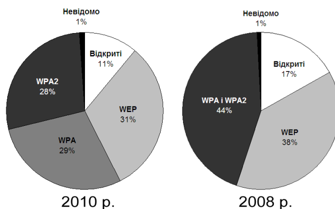
Рис. 1.27. Діаграма шифрування ТБД у відсотках за 2008 і 2010 рр.
